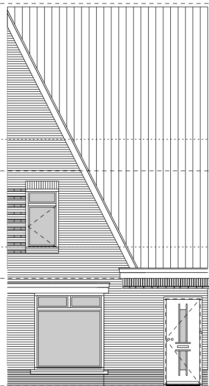
voorgevel 5400
